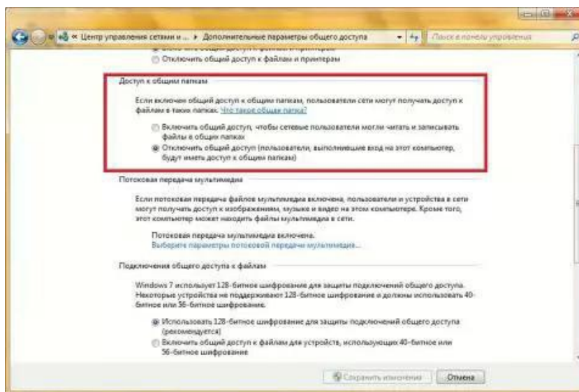
Рис.182.Отключениеобщегодоступаппакпке «Общие»
