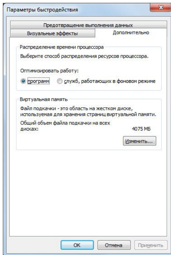
Рис.84.Параметрыбыстродей- ствия
