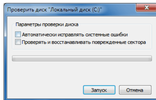
Рис.32. Параметры проверки
